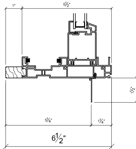
5 1/4" JAMB
